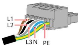
Borne del lado del inversor (trifásico)
