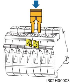
Borne de CA para la red eléctrica (X2) (monofásico/trifásico)
