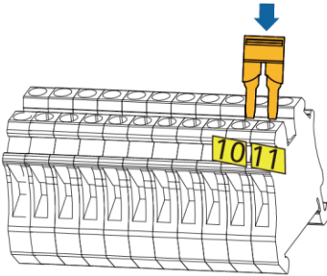
Borne de CA X3 del inversor (monofásico)
