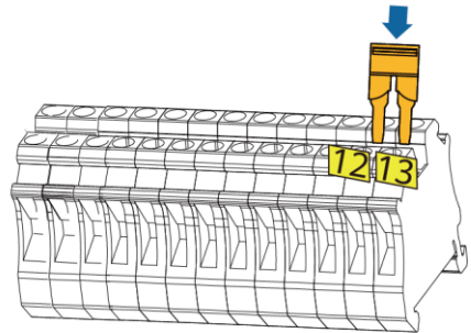
Borne de CA X3 del inversor (trifásico)
