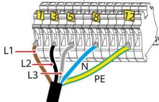
Borne del lado del Backup Box (trifásico)
