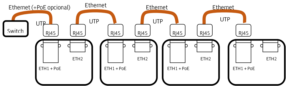
Conexión encadenada de varios terminales
