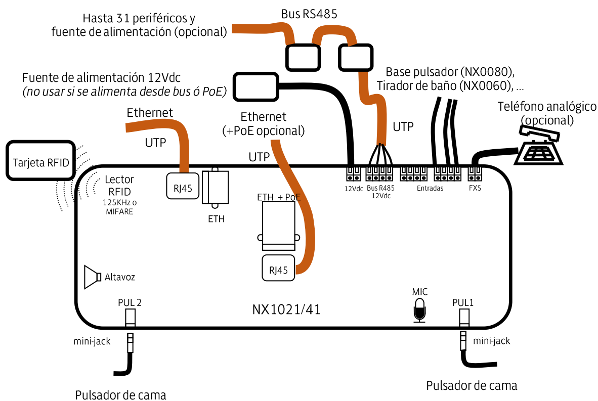
Cableado de NX1021/41
