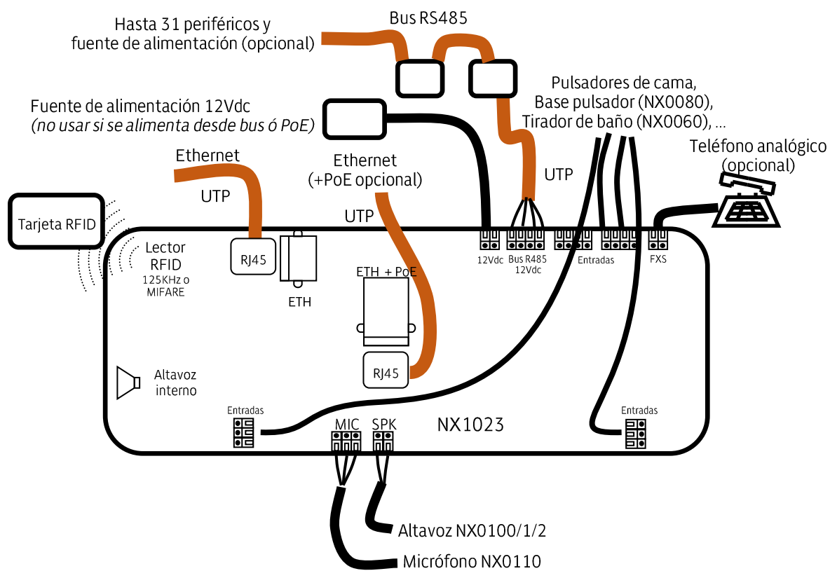
Cableado de NX1023
