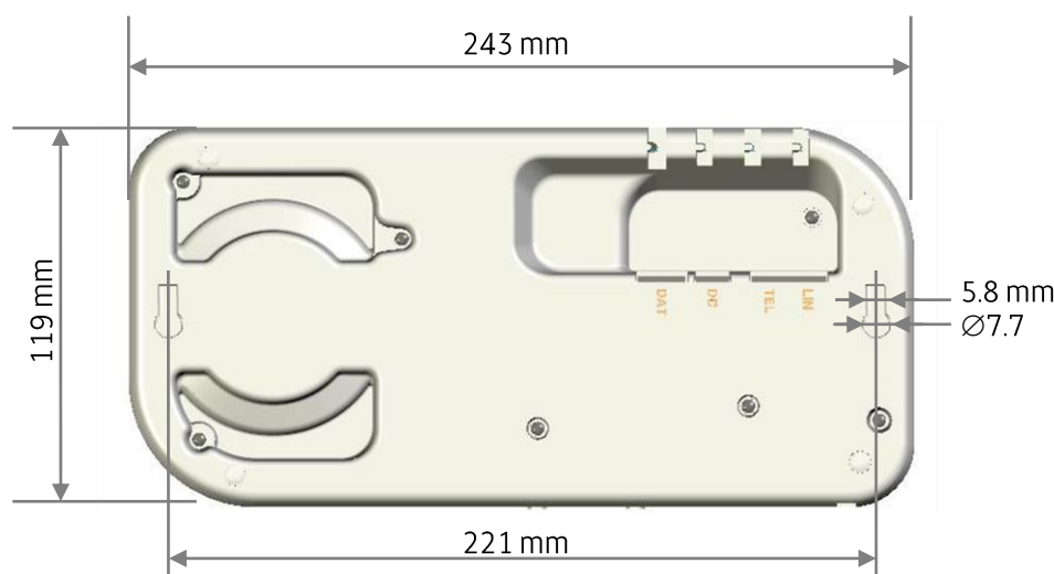
Dimensiones de NX0017/18/19/19V2(D)(B)
