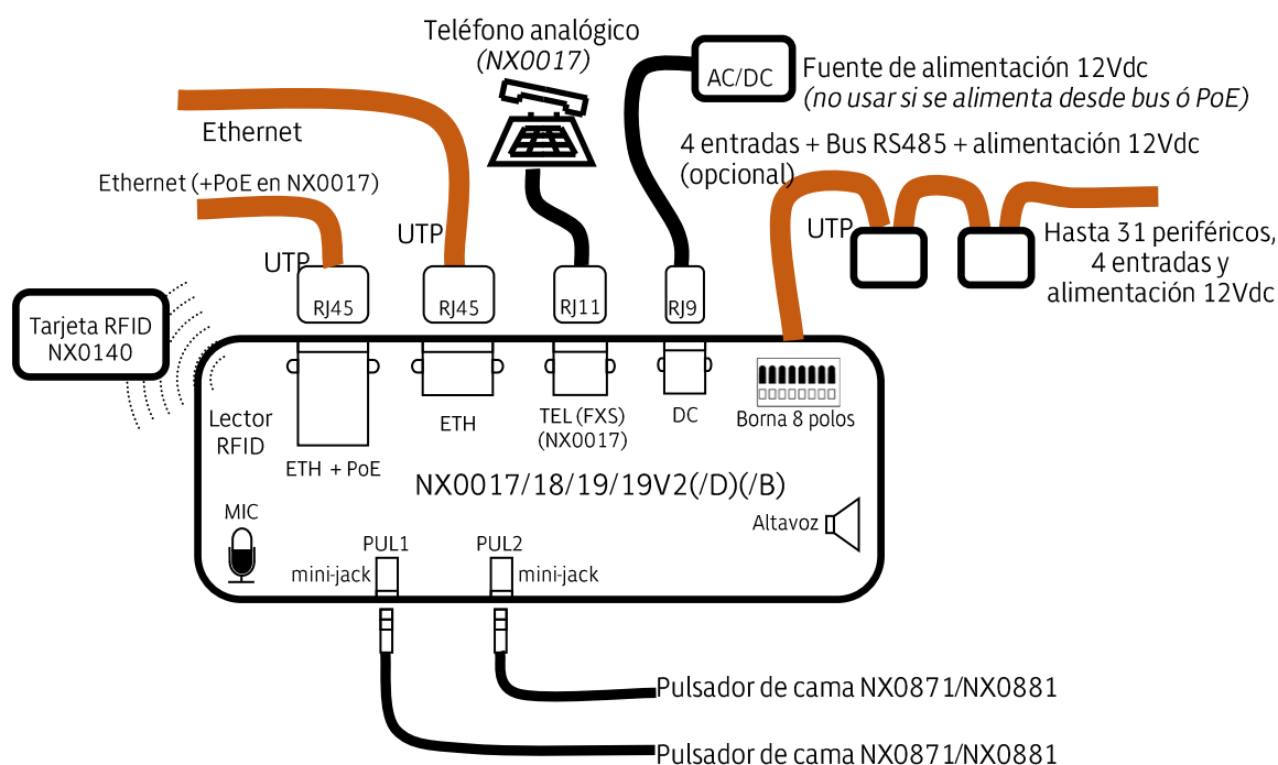
Cableado de NX0017/18/19/19V2(D)(B)
