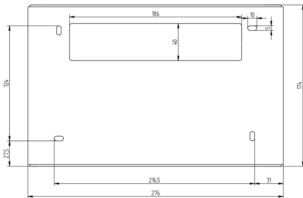
Dimensiones carcasa trasera NX1041
