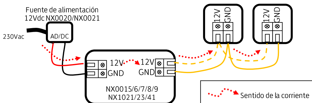
Alimentación de dispositivos utilizando una fuente de alimentación
