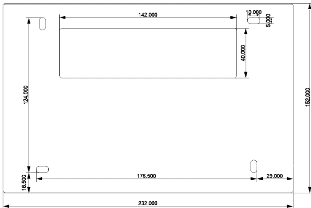
Dimensiones carcasa trasera NX1021
