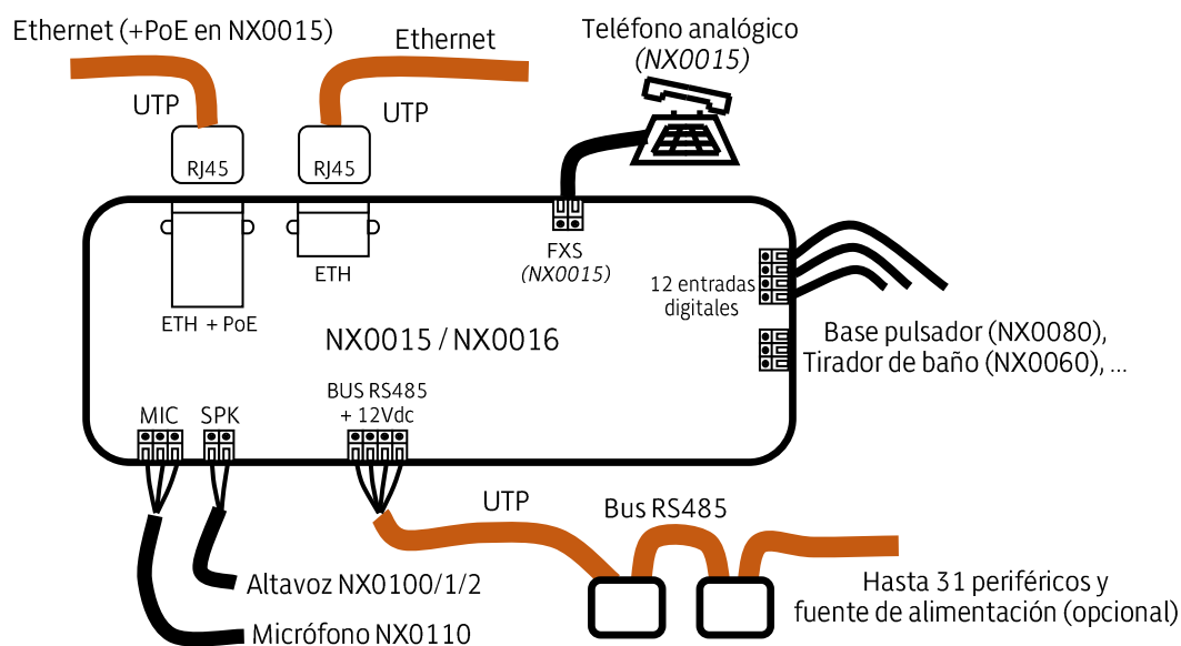
Cableado de NX0015/6
