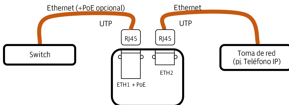
Conexión de una toma de red a la boca ETH2
