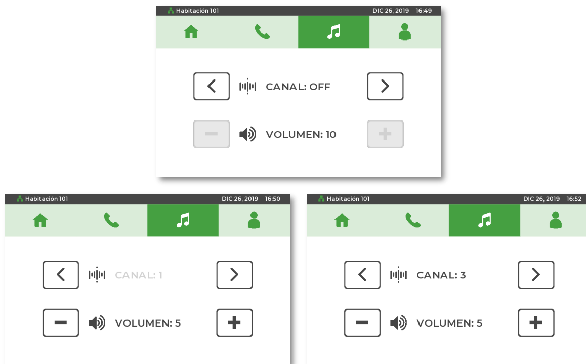
Menú Megafonía sin canal seleccionado, con canal 1 inactivo y con canal 3 activo
