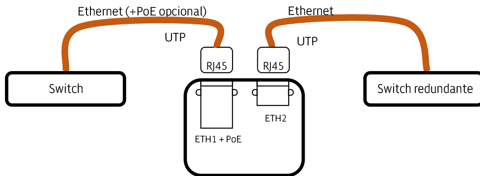
Conexión de Ethernet redundante
