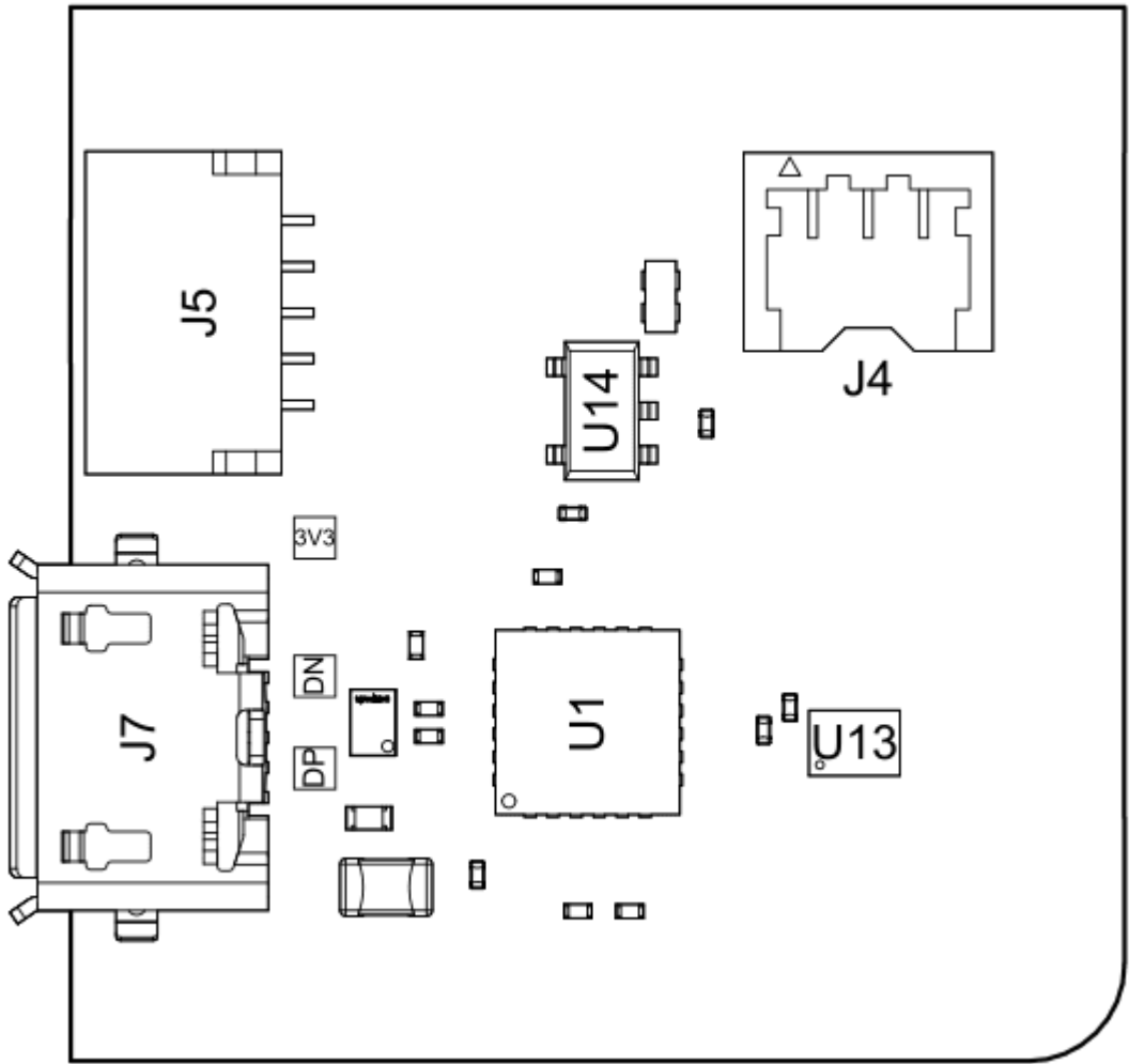
电路板背面视图
