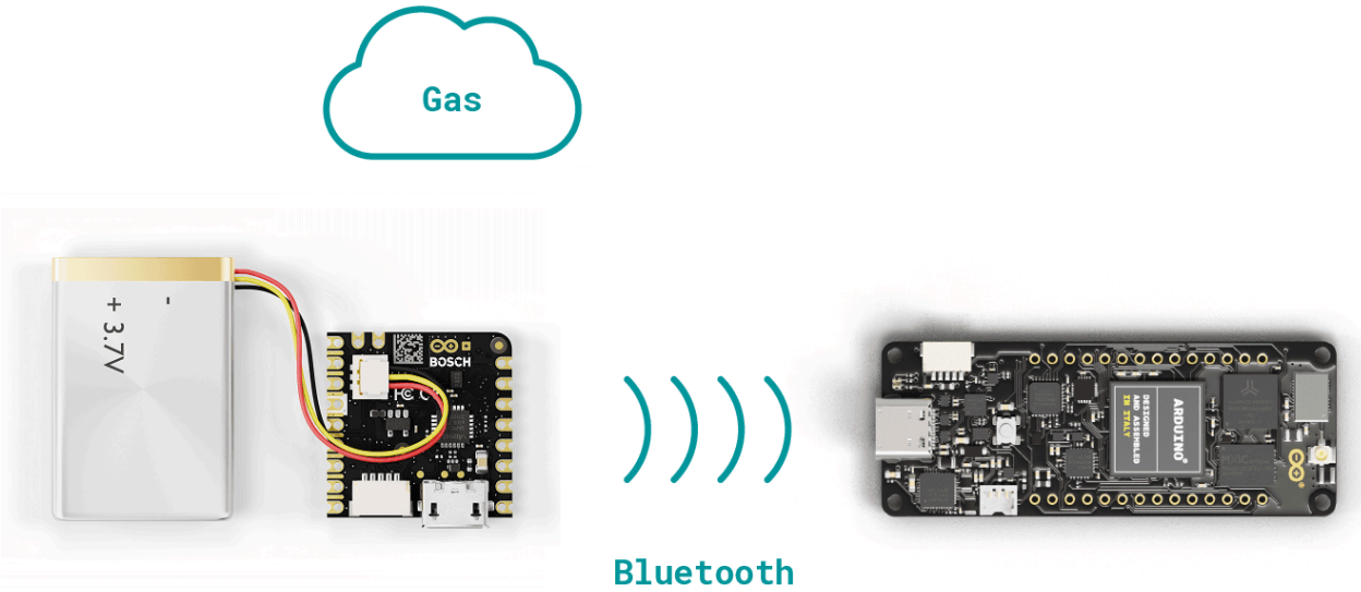
远程环境监测的典型解决方案示例，包括Arduino® Nicla Sense ME、Portenta H7和电池。请注意电池电缆在电路板连接器中的方向。
