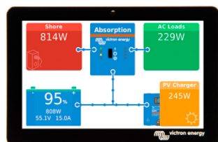
GX Touch (pantalla opcional para Cerbo GX y Cerbo-S GX)
