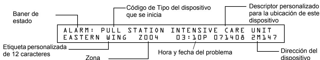
Figura 3.2 Ejemplo de pantalla de alarma de incendios
