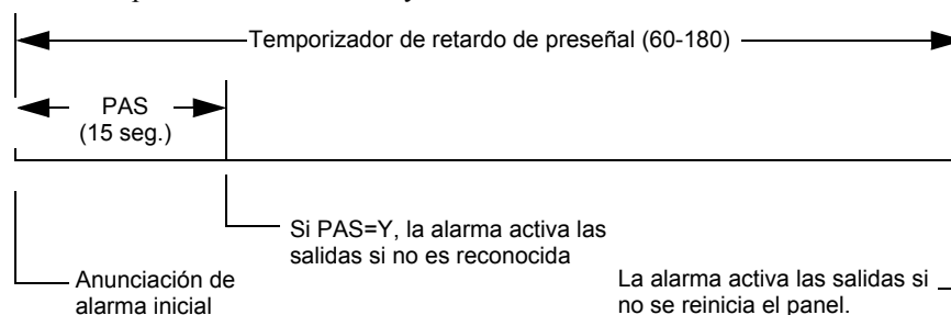
Figura A.7 Tiempo de preseñal y PAS
