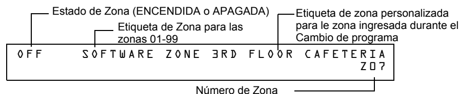
Figura 4.4 Pantalla de Ejemplo de Estado de Lectura de la Zona de Software
