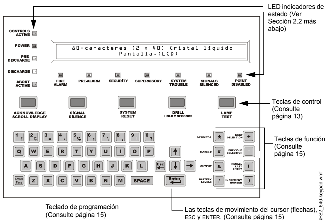
Figura 2.1 Teclas e indicadores del panel de control NFS2-640
