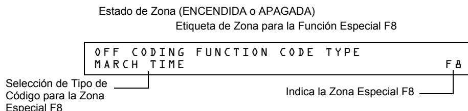
Figura 4.5 Pantalla de Ejemplo de Estado de Lectura de la Zona Especial
