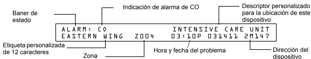
Figura 3.12 Ejemplo de pantalla de alarma de CO
