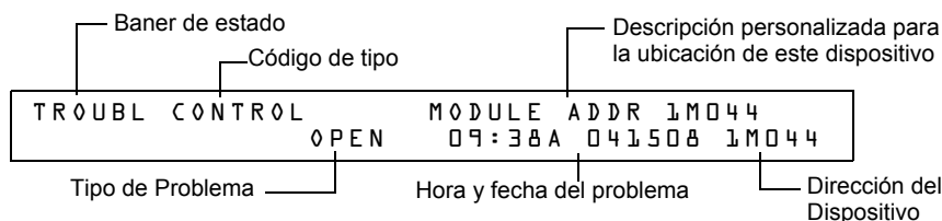
Figura 3.16 Ejemplo de Mensaje de Problemas en Módulo de Relé/Control
