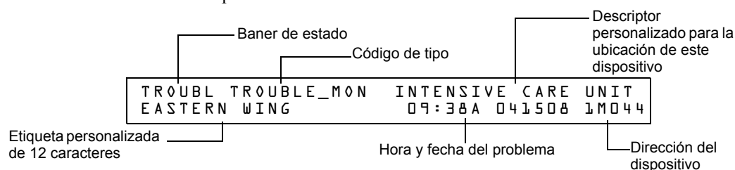
Figura 3.14 Ejemplo de Problema Mensaje de Punto de Monitor
