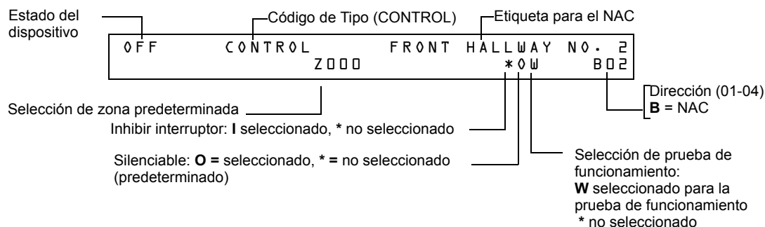
Figura 4.3 Pantalla de Ejemplo de Estado de Lectura del NAC
