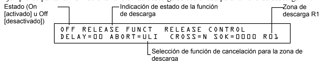
Figura A.1 Ejemplo de Read Status (estado de lectura) para una zona de descarga
