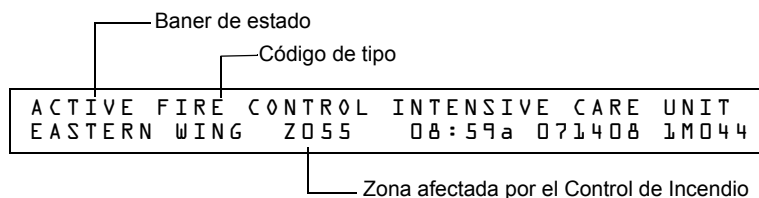
Figura 3.11 Pantalla de Punto de control de Incendio
