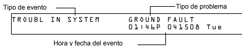
Figura 4.17 Pantalla de ejemplo de Evento de Problema
