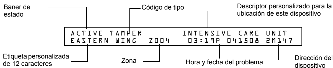
Figura 3.8 Mensaje de Muestra de Señal de Supervisión
