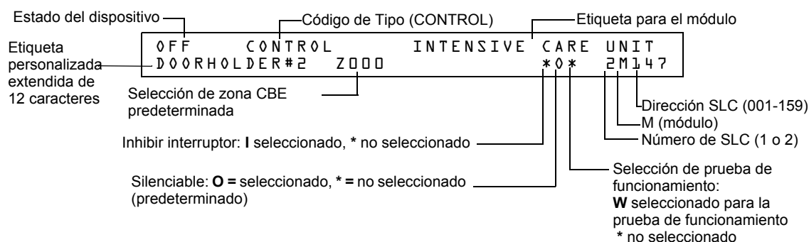
Figura 4.2 Ejemplo de Pantalla el Estado de Lectura del Relé/Control o del Módulo de Monitor
