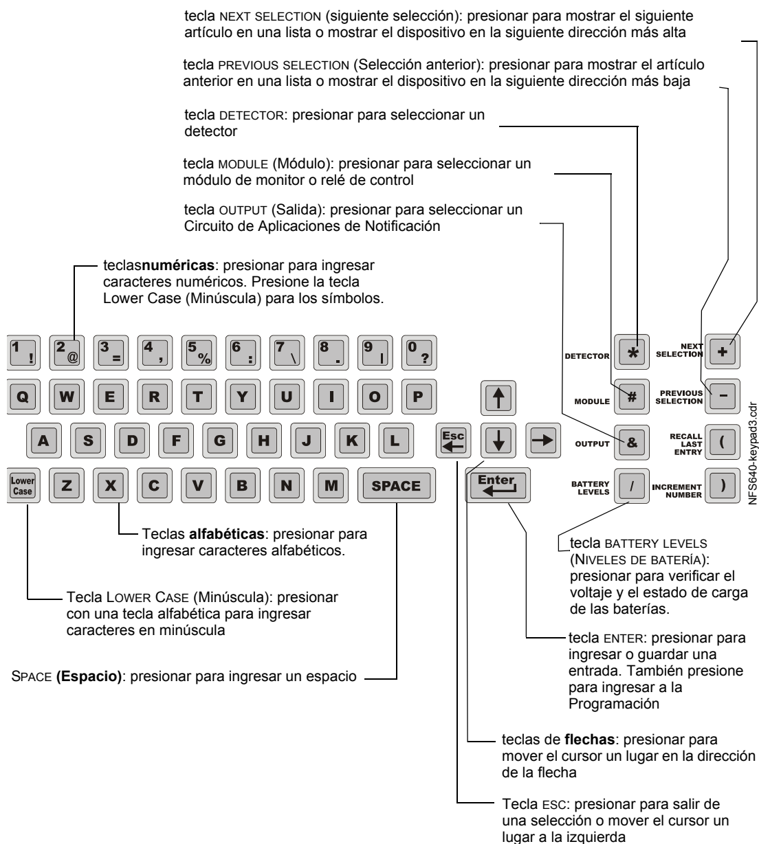
Figura 2.2 Teclado de programación
