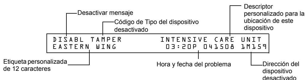
Figura 3.10 Ejemplo del mensaje de Punto Desactivado
