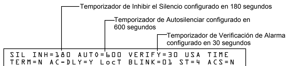
Figura 3.17 Pantalla de ejemplo de selección de función del sistema
