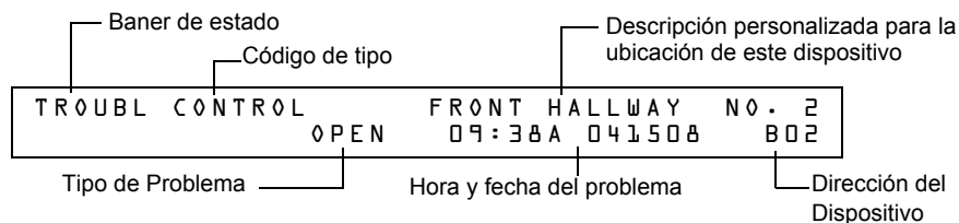
Figura 3.15 Ejemplo de Mensaje de un NAC en Problemas
