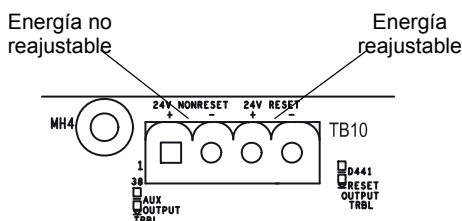
Figura 3.16 Salidas de la fuente de energía de CC - TB10
