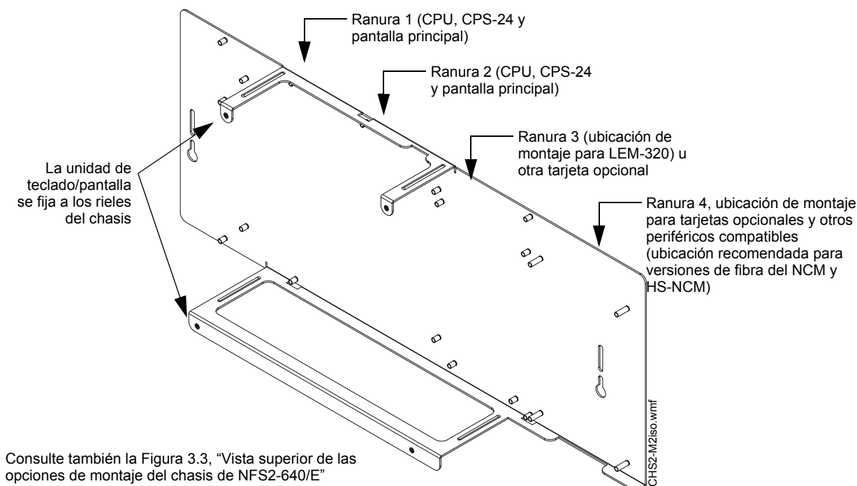
Figura 3.2 Vista lateral de las opciones de montaje del chasis de NFS2-640/E
