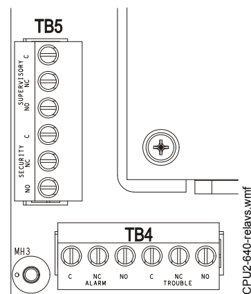
Figura 3.21 Conexiones del relé forma C
