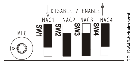
Figura 3.22 Interruptores de la alarma de respaldo
