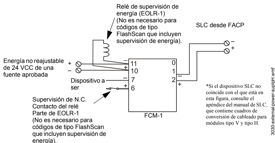
Figura 4.1 Activación de supervisión de energía externa utilizando relés
