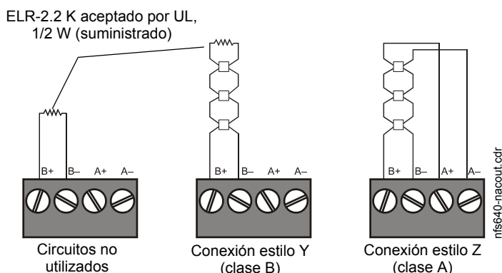
Figura 3.18 Conexiones del circuito de dispositivo de notificación (NAC)
