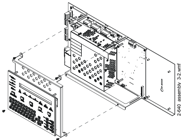
Figura 3.5 Montaje de KDM-R2
