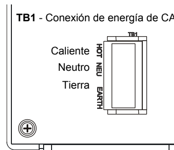
Figura 3.14 CPS-24/E: Conexiones de energía de CA
