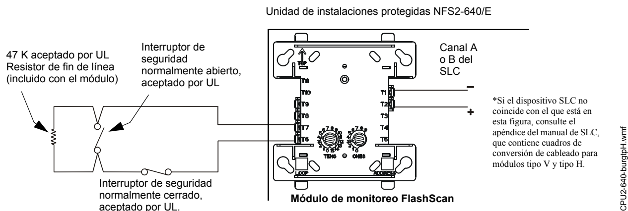
Figura 4.6 Diagrama de cableado para aplicaciones de alarma de seguridad patentadas
