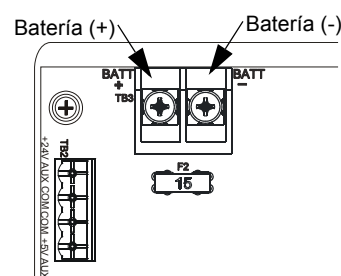
Figura 3.15 CPS-24/E: Conexiones de energía de CC
