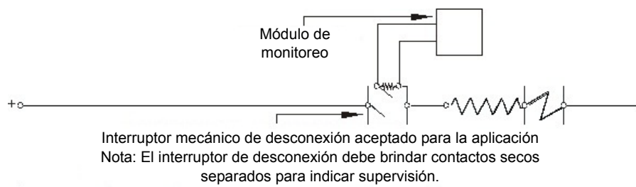
Figura 4.11 Circuitos de descarga (interruptor mecánico de desconexión)
