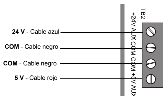
Figura 3.17 Conexión a la salida de los accesorios TB2 en CPS-24/E
