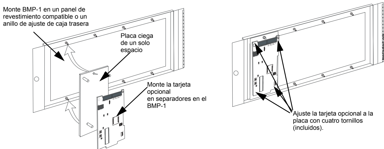
Figura 3.10 Montaje de una tarjeta opcional sobre un panel de revestimiento con BMP-1 (se muestra ADP-4B)
