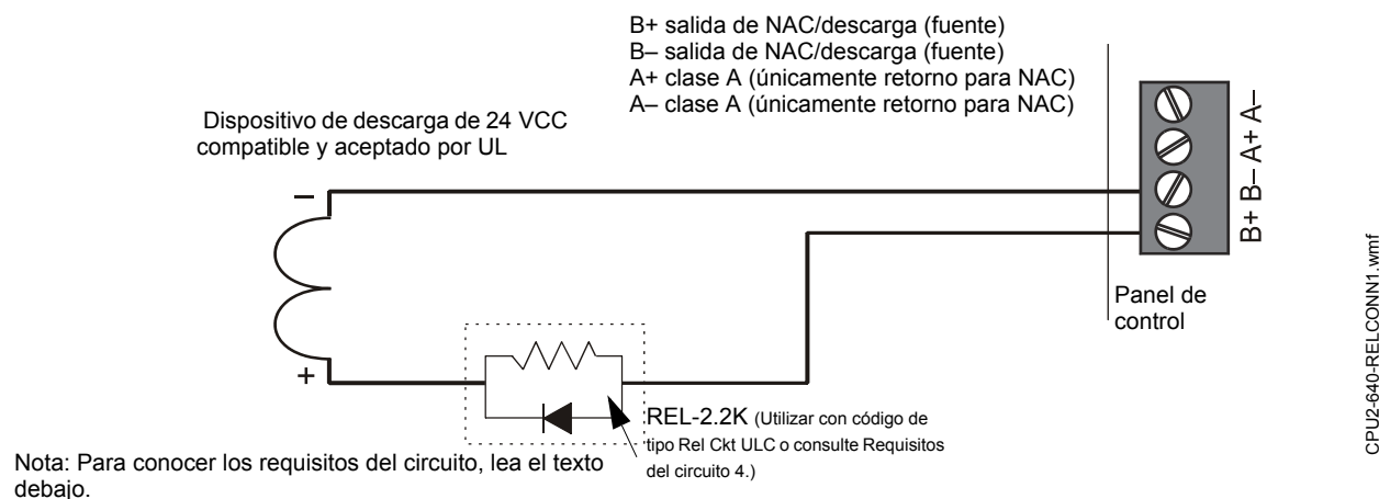
Figura 4.7 Conexión estilo 4 típica de un dispositivo de descarga al panel de control
