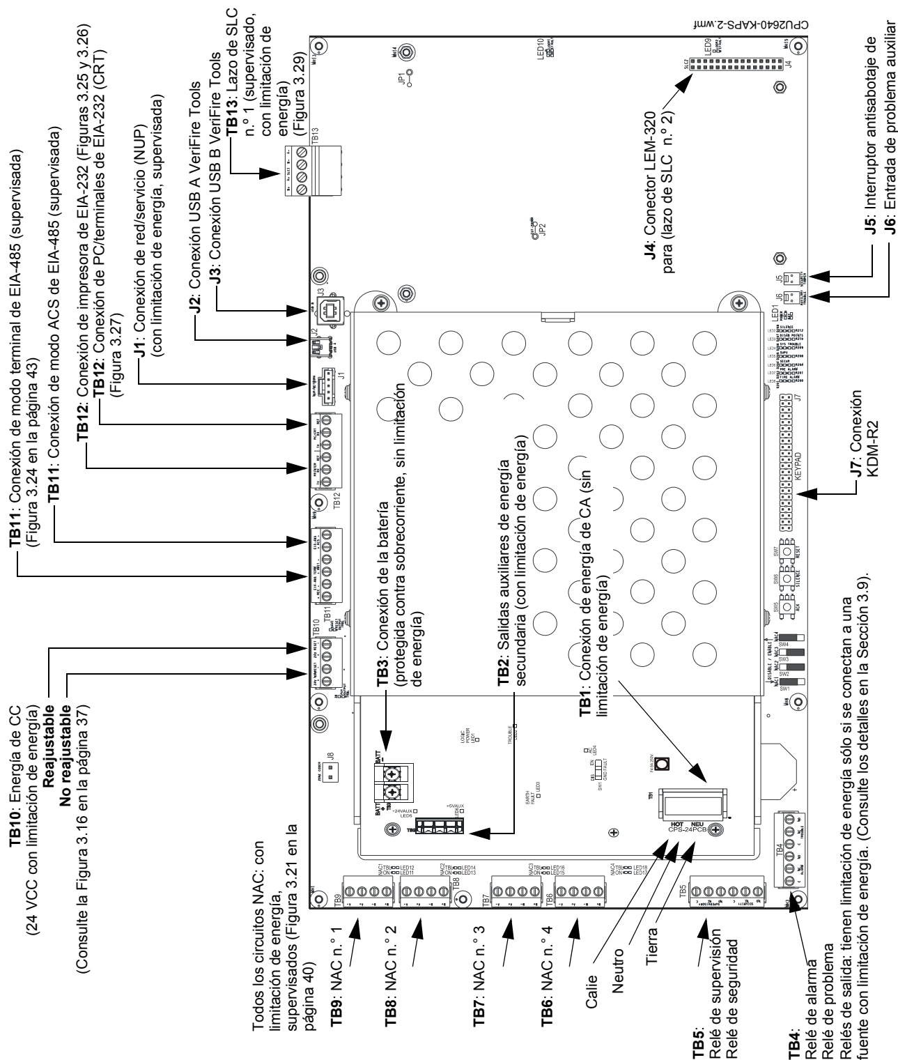
Figura 2.2 CPU2-640/CPU2-640E y fuente de energía: Conexiones eléctricas
