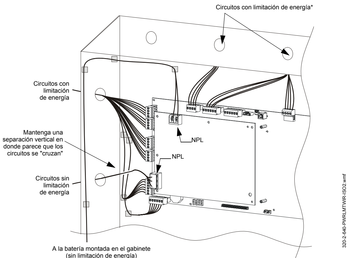
Figura 3.23 Cableado típico que cumple con los requisitos de UL para el cableado con limitación de energía (Se muestra con relés conectados a módulos con limitación de energía)
