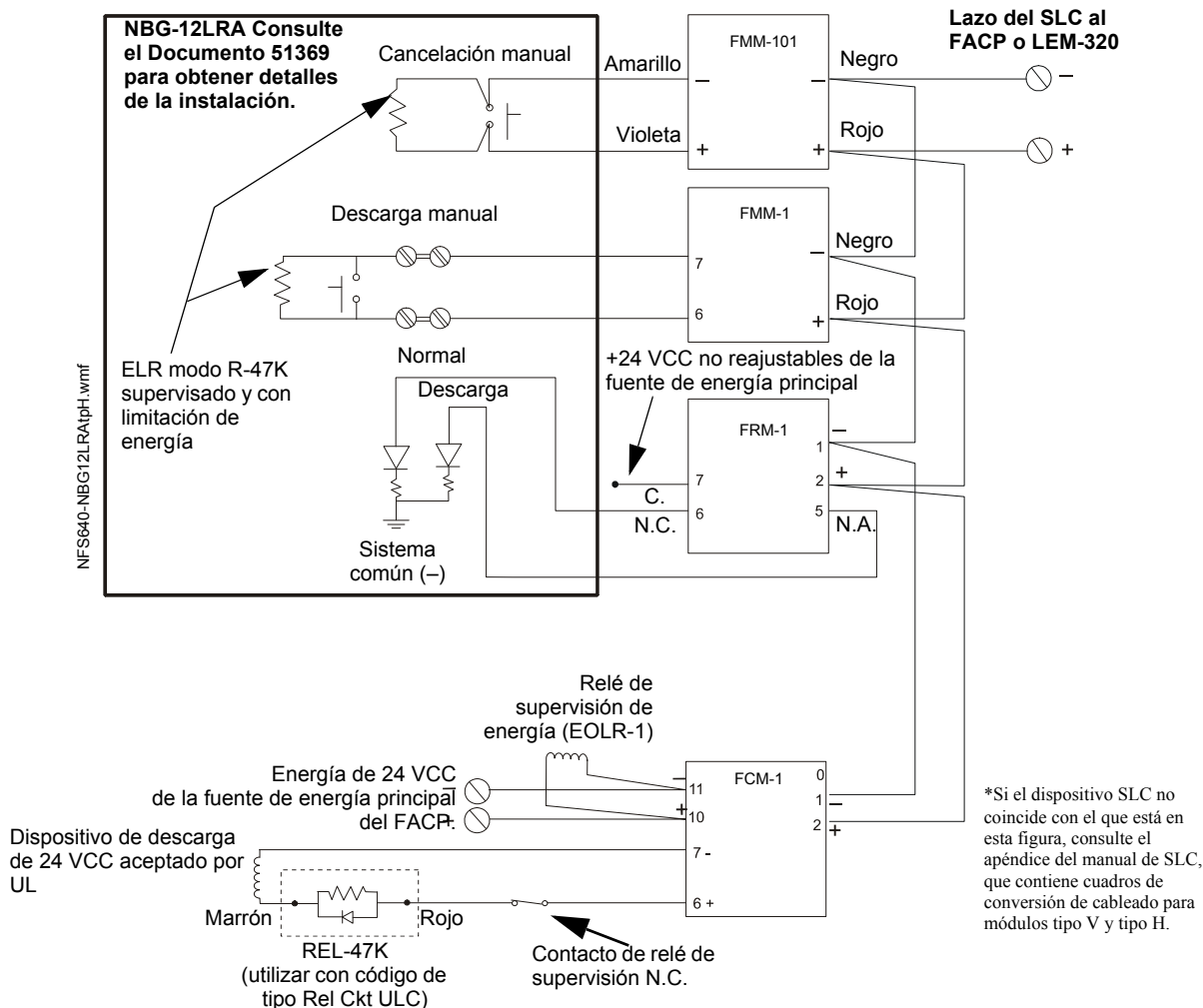
Figura 4.14 Conexión típica para una estación de descarga-cancelación del agente NBG-12LRA
