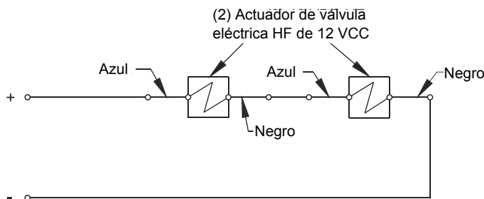
Figura 4.9 Circuitos de descarga (opción 2)
