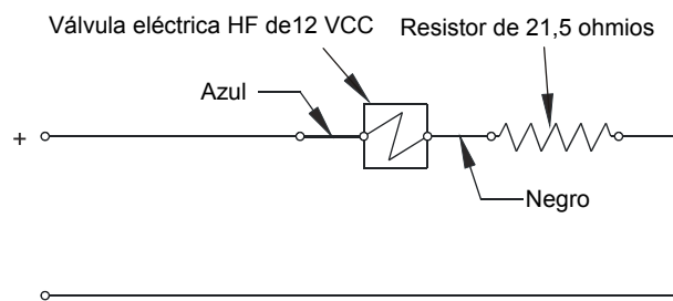
Figura 4.10 Circuitos de descarga (opción 3)
