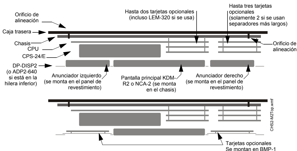
Figura 3.3 Vista superior de las opciones de montaje del chasis de NFS2-640/E
