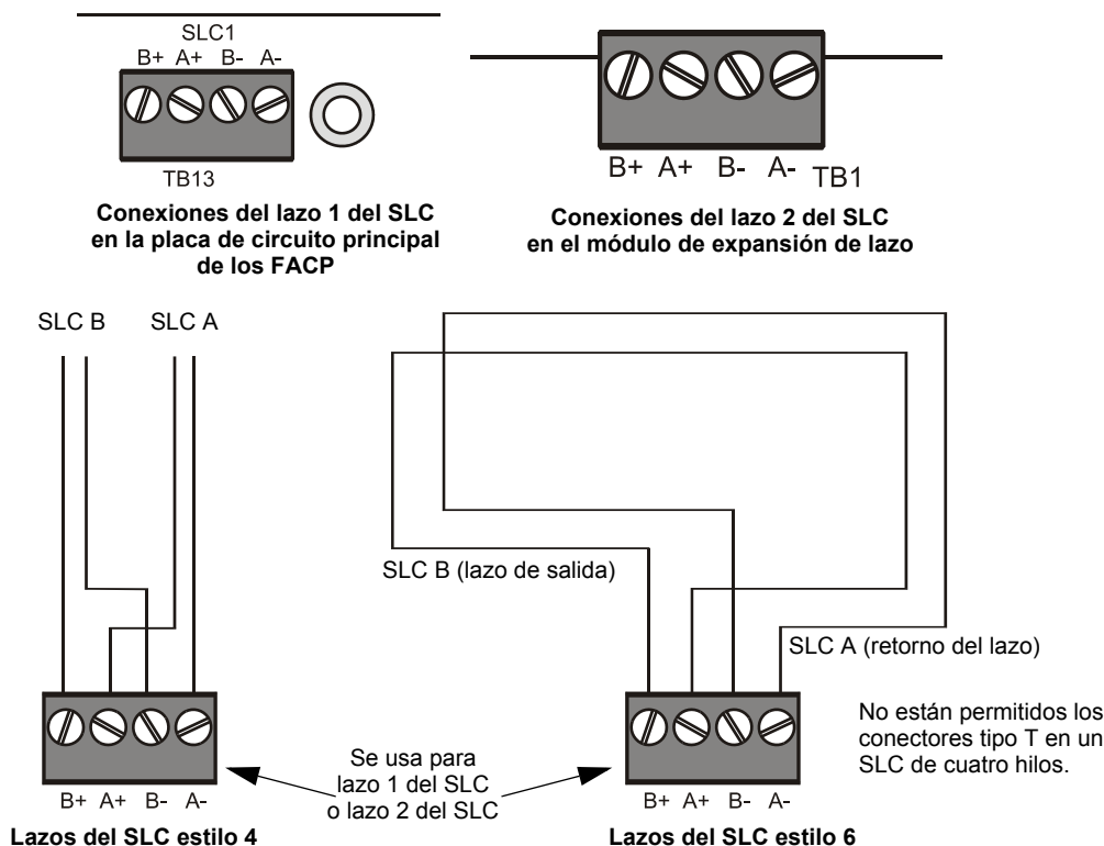
Figura 3.29 Conexiones y cableado del lazo del SLC
