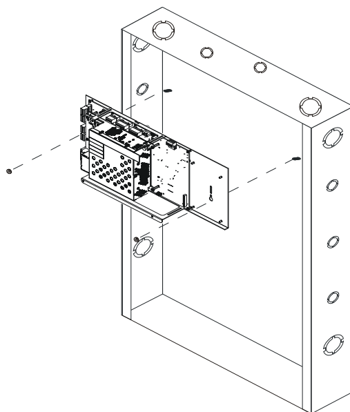
Figura 3.4 Montaje del chasis de NFS2-640/E
