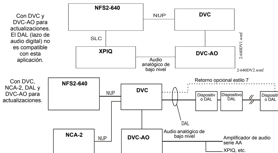
Figura 3.13 Diagramas de bloques de aplicaciones de la serie DVC
