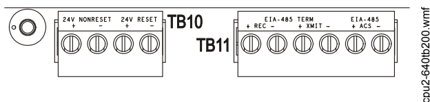
Figura 3.24 Conexiones de EIA-485
