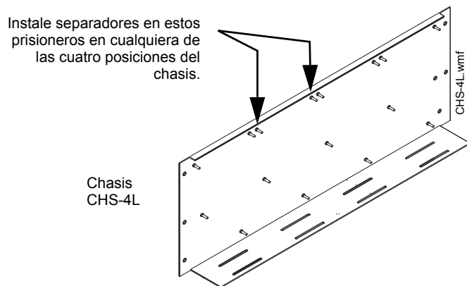
Figura 3.8 Ubicaciones de los separadores en CHS-4L
