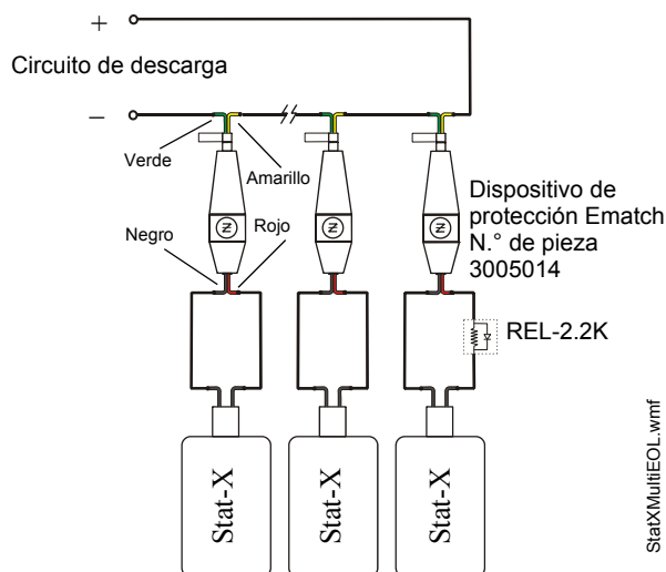
Figura 3.20 Diagrama de cableado para dispositivos Stat-X
