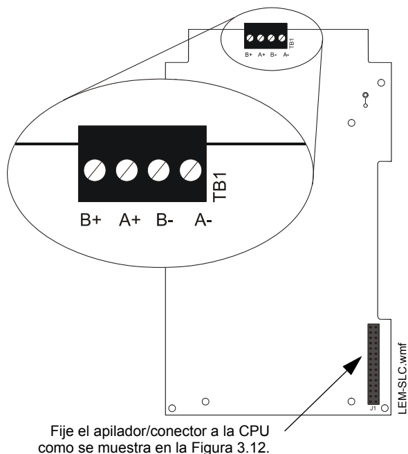
Figura 3.11 Conexiones de SLC para LEM-320
