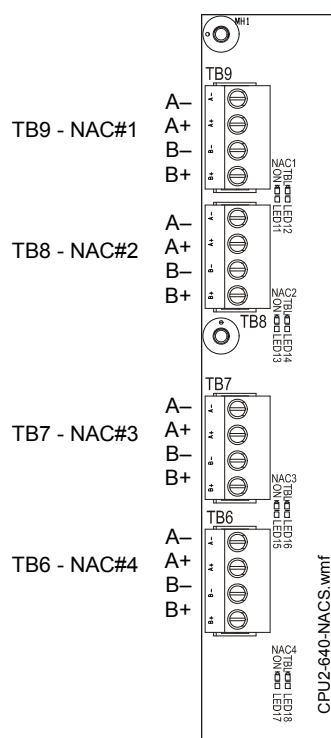
Figura 3.19 Terminales y LED del NAC
