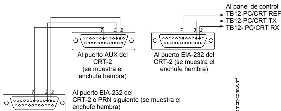
Figura 3.28 Conexión de varios dispositivos en el circuito EIA-232
