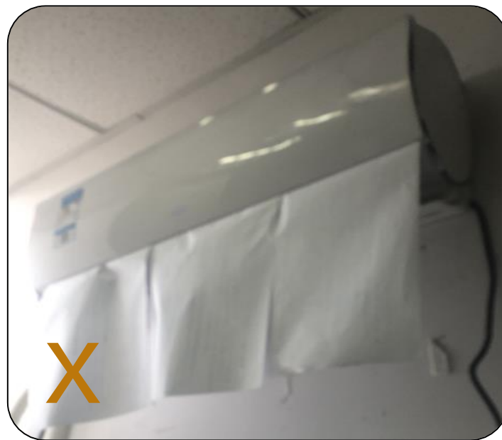
Instalación incorrecta Salida del Aire bloqueada.
